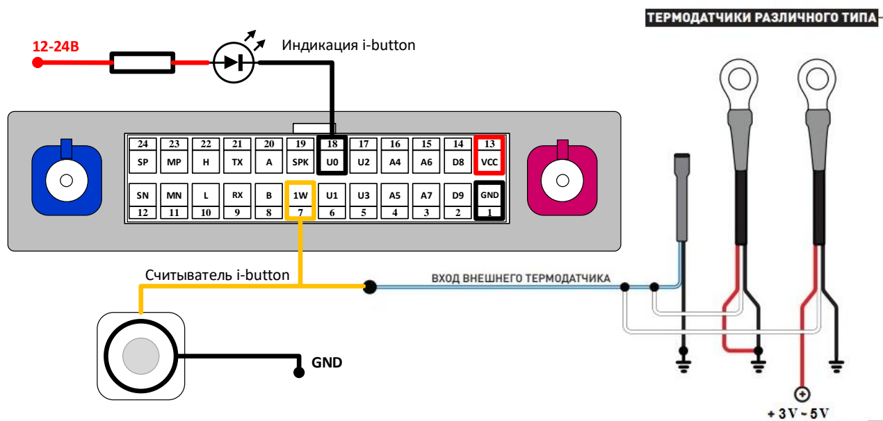
Рисунок 8 – Схема подключения термодатчиков различного типа
